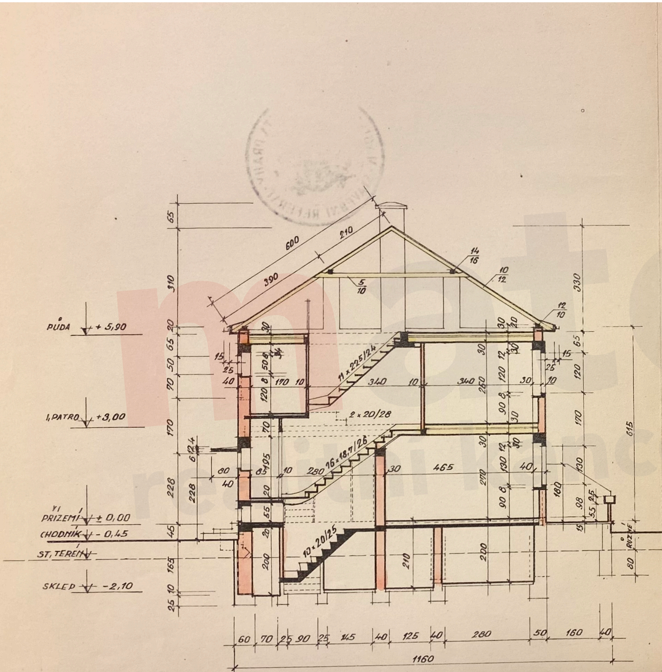
PRÍČNÝ ŘEZ SCHODÍSTĚM.
